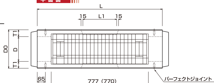
平面図
