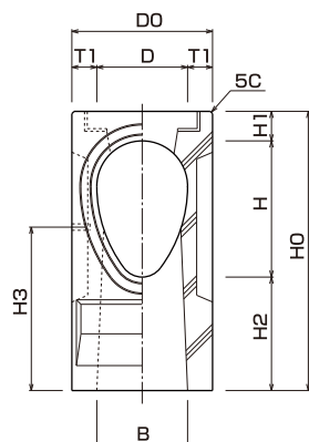
寸法表
