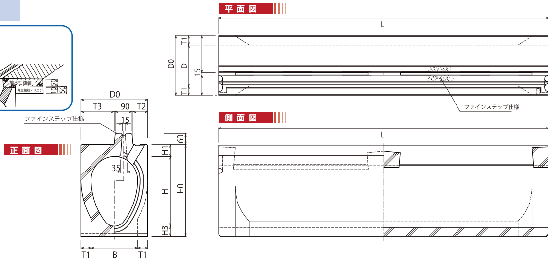
寸法表
