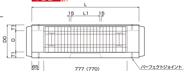
平面図
