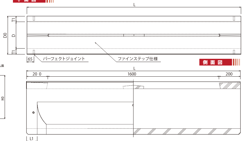
平面図
