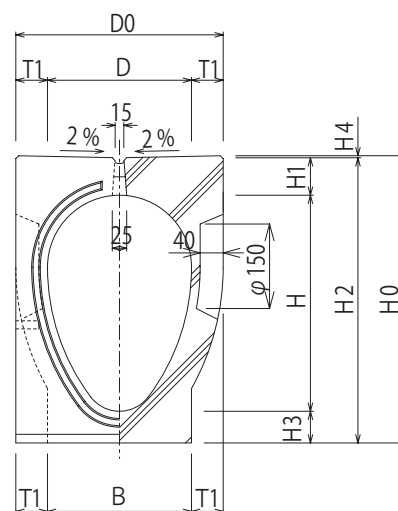
正面図
