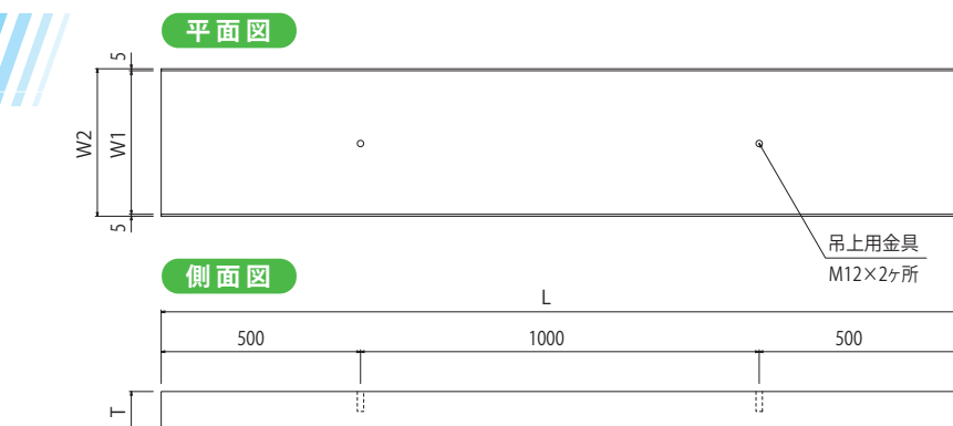
寸法表
