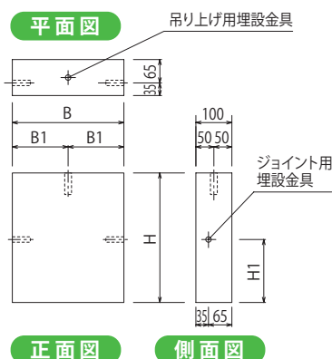
寸法表
