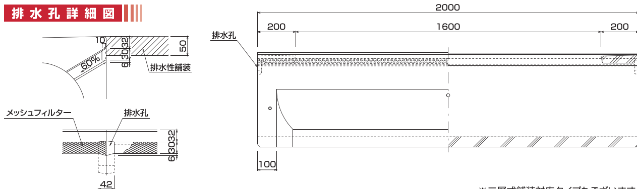
側面図
