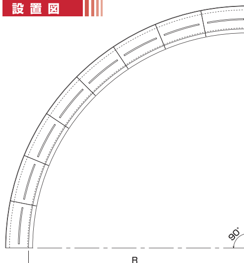
設置図
