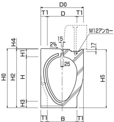
正面図
