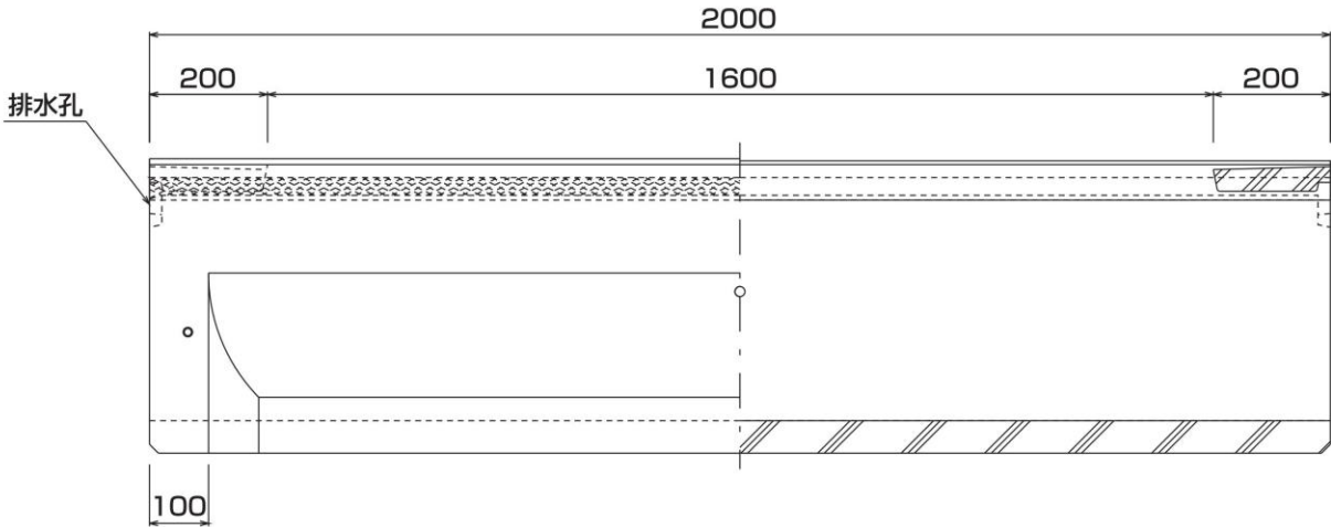
側面図
