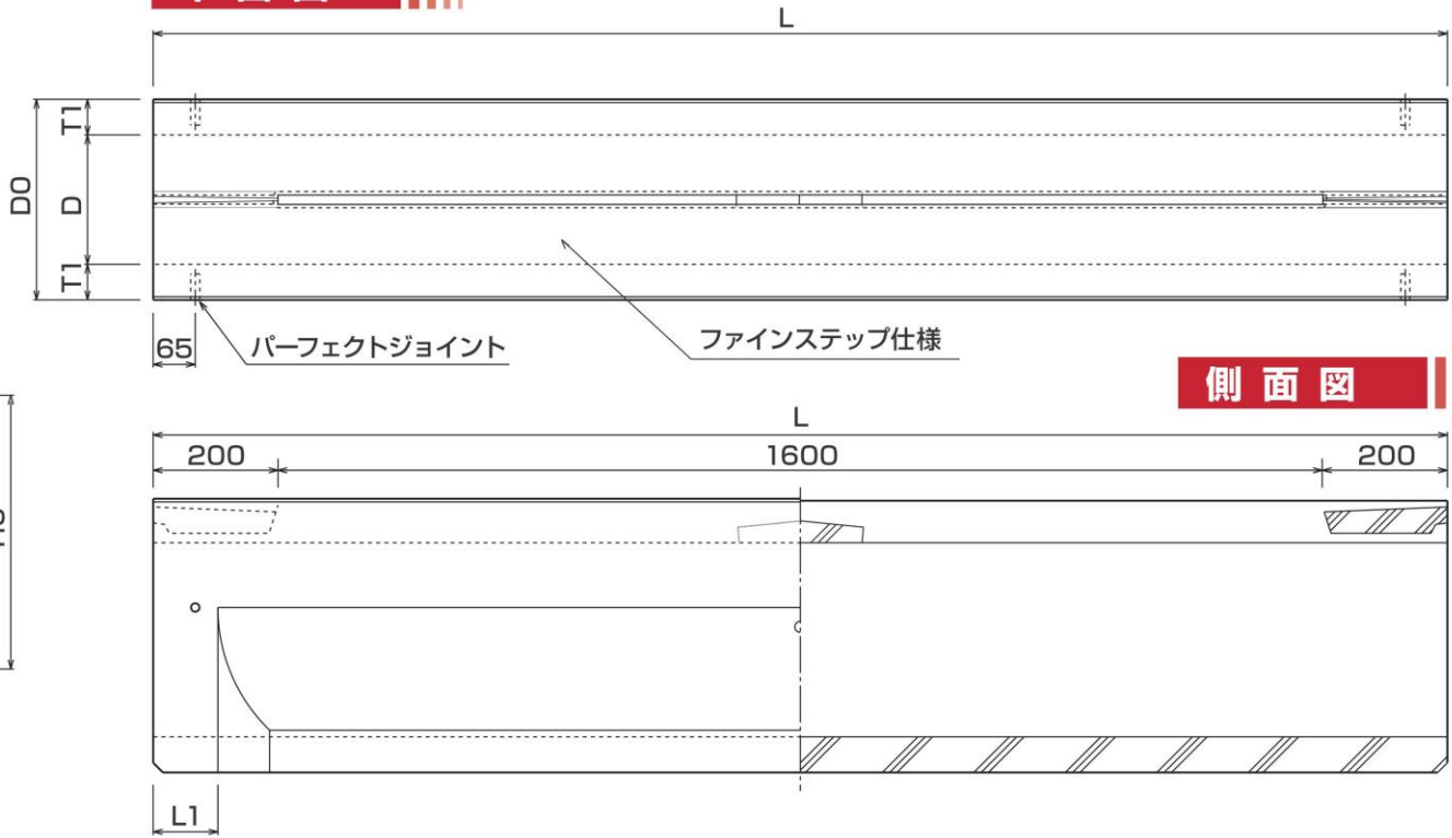
平面図
