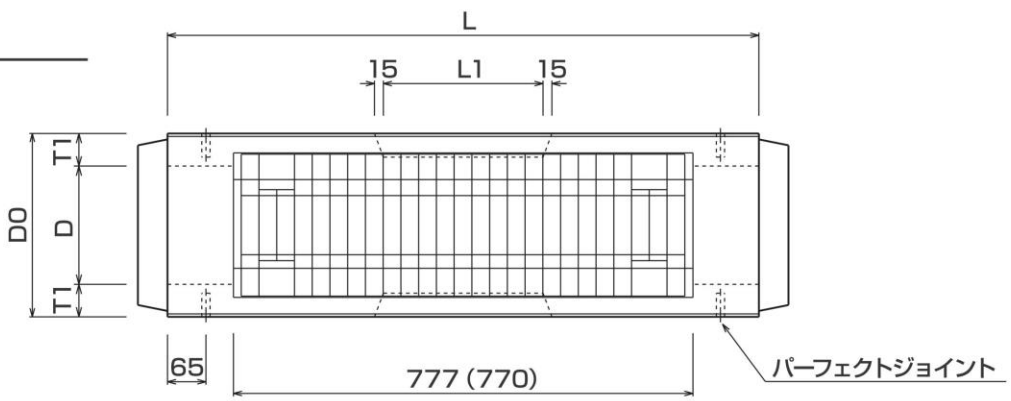
平面図
