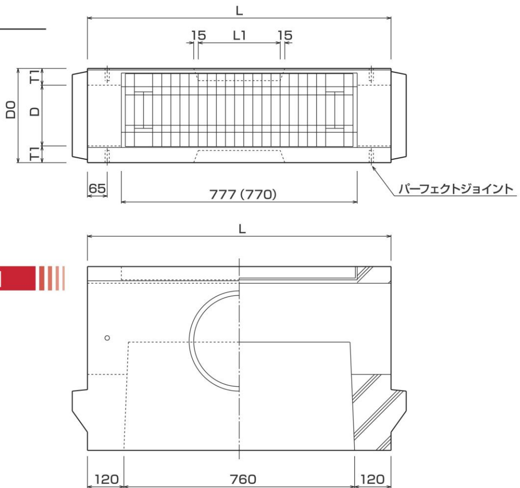
側面図
