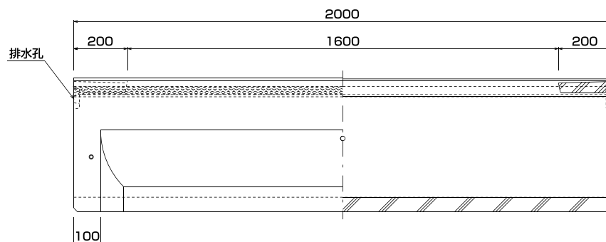
側面図
