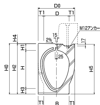
正面図
