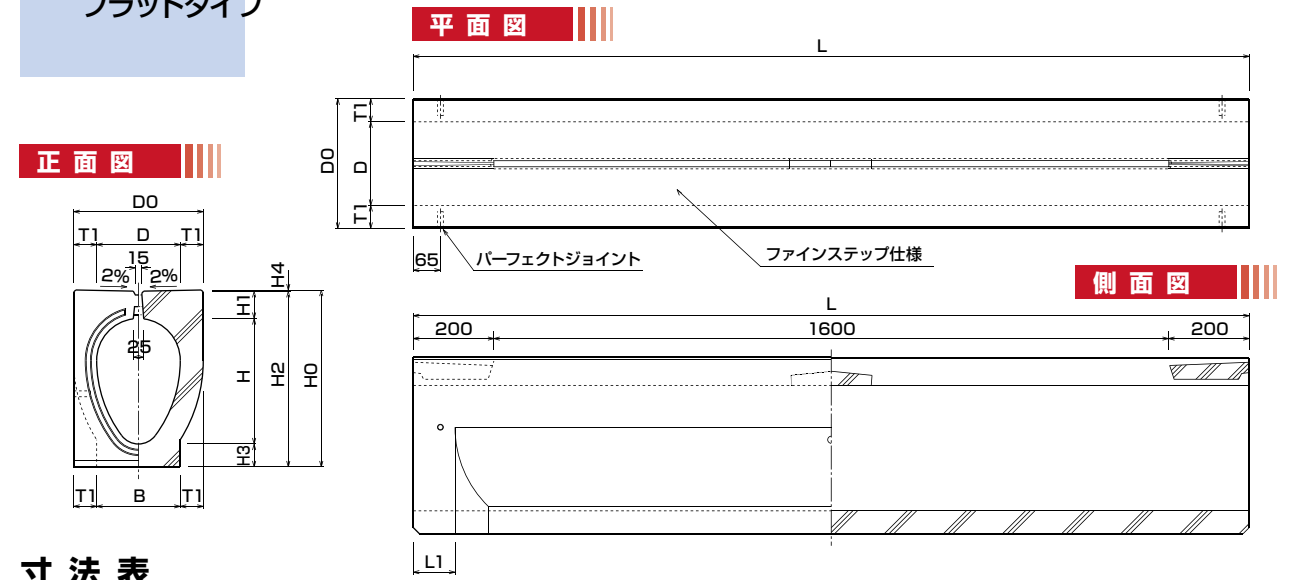
寸法表
