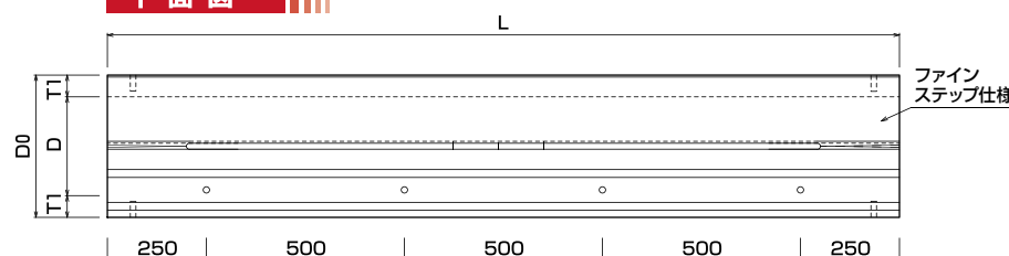
側面図
