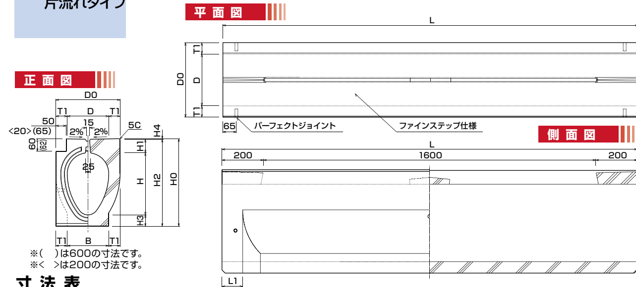
寸法表
